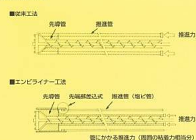
図1. 推力伝達機構の比較
